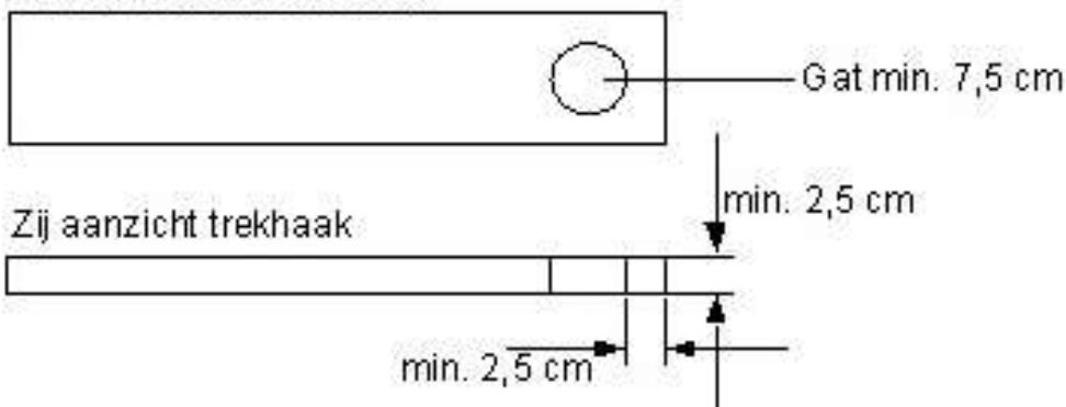
Boven aanzicht trekhaak
